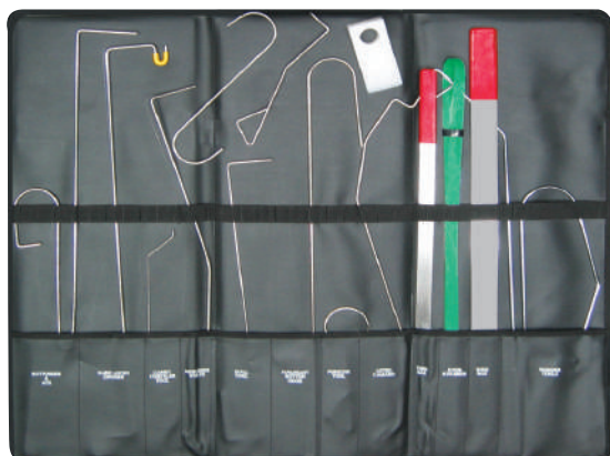
UT186K 17 PCS. Deluxe Universal Lockout Tool Set Outils Universels de Déverrouillage
